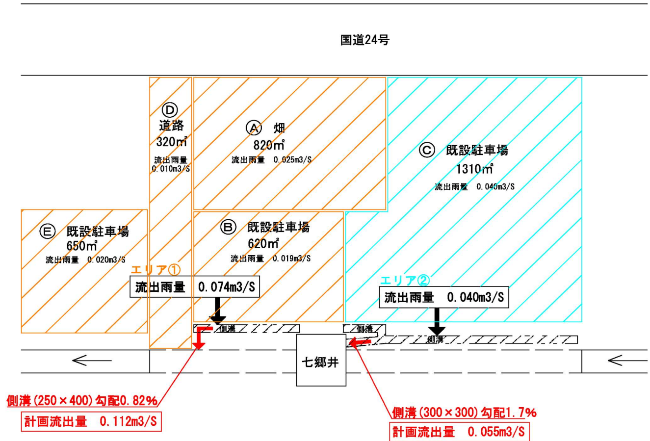
平面図
