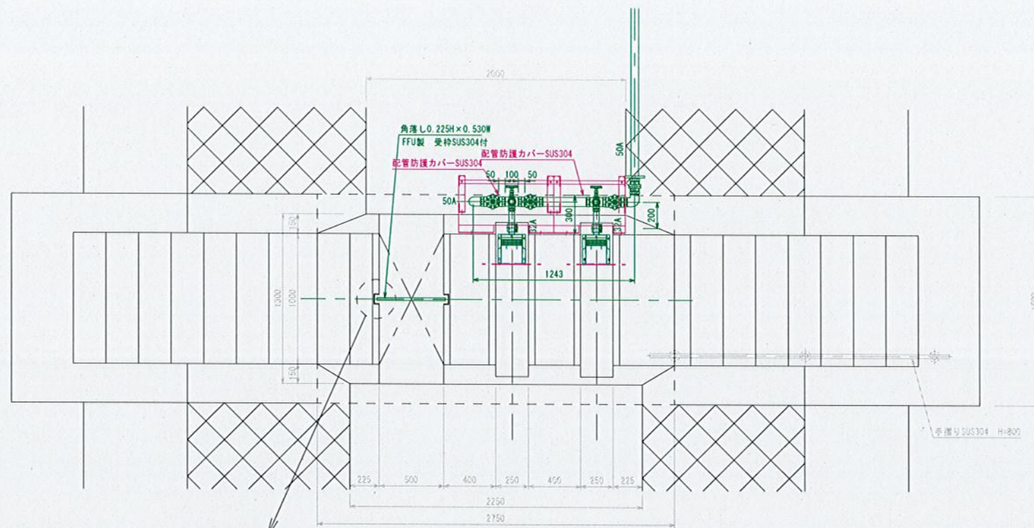
平面図 S=1/20
