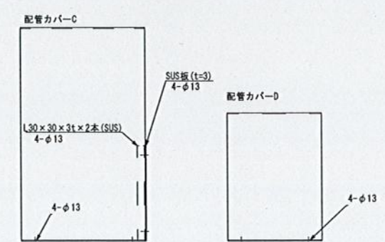
側面図
