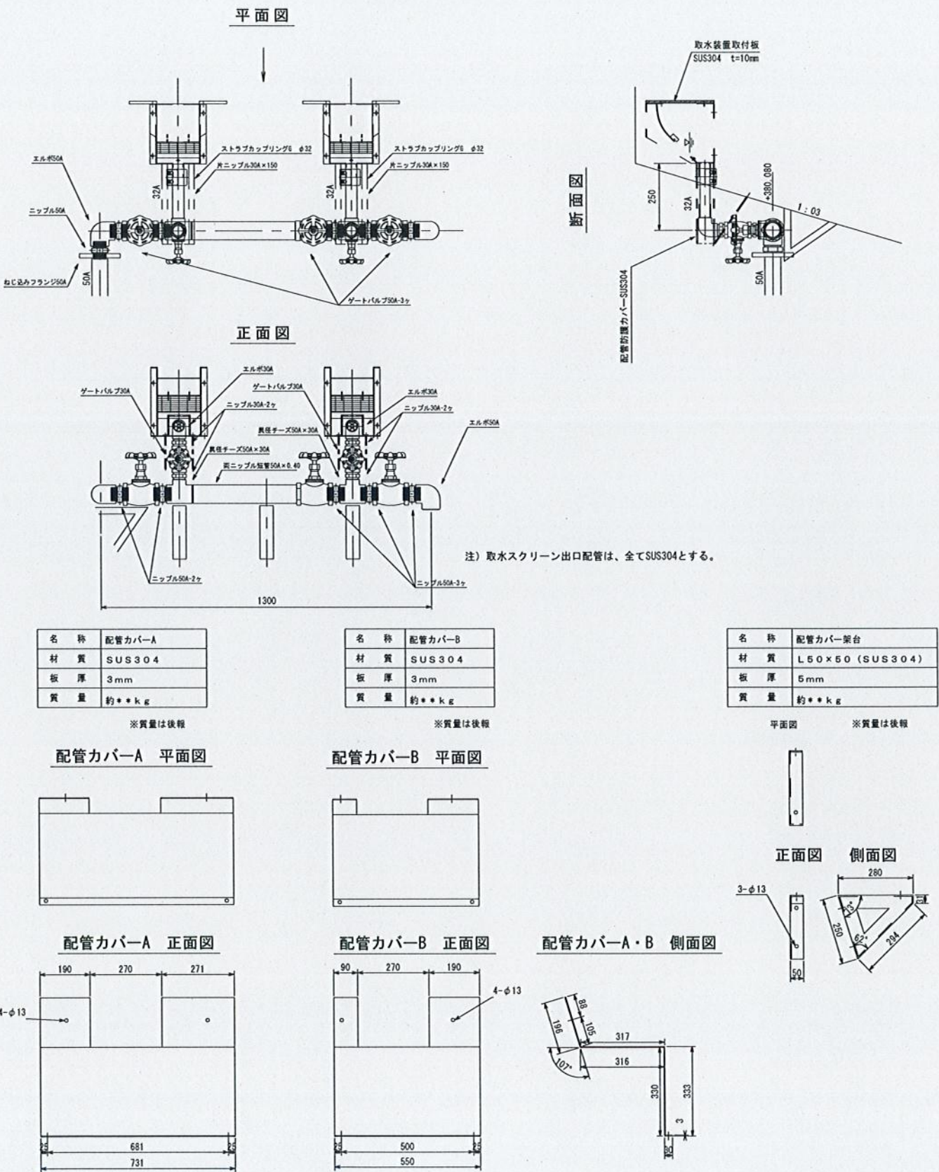
取水配管詳細図 S=1/10
