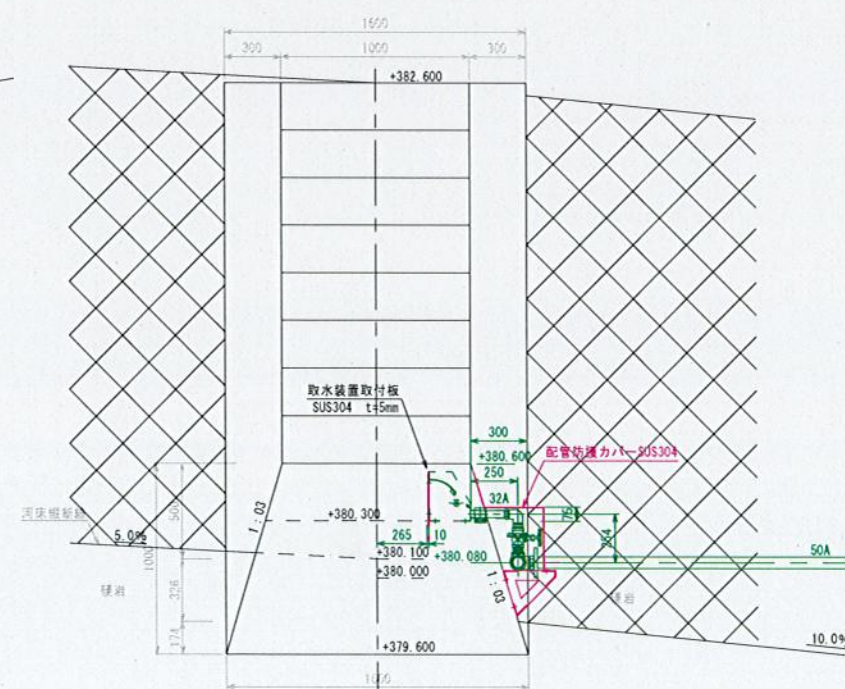
縦断図 S=1/20
