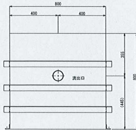
沈砂槽廻り配管詳細図
