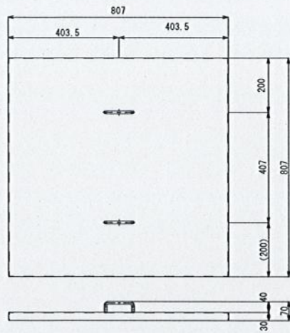
背面図 (流出部)
