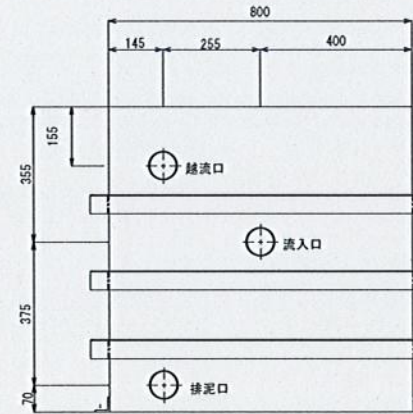
正面図 (流入部)
