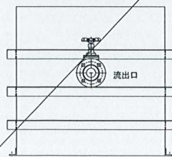
背面図 (流出部)
