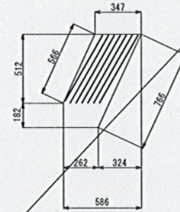
側面図
