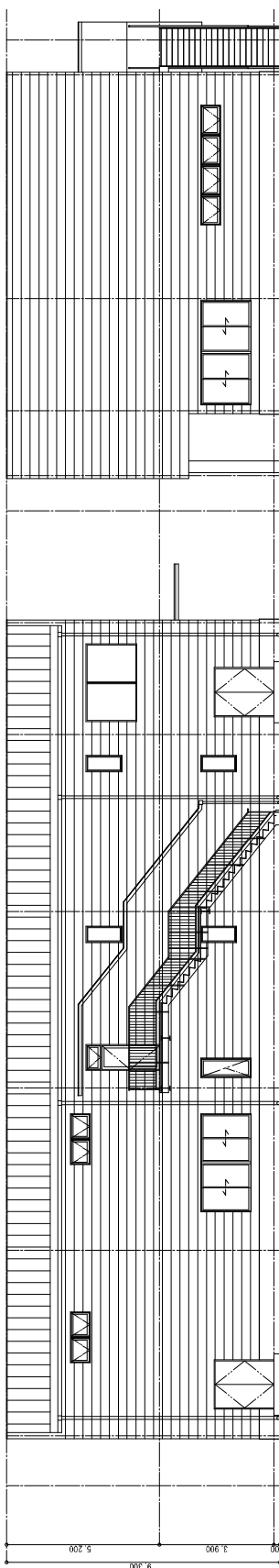
东侧立面图
