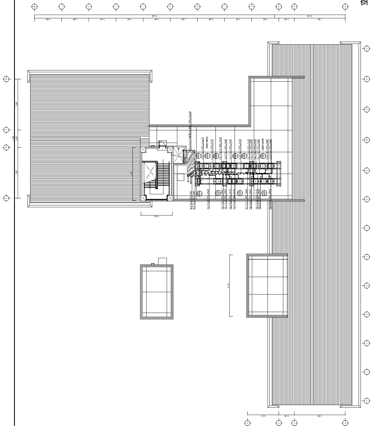
空調設備 R 階平面図
